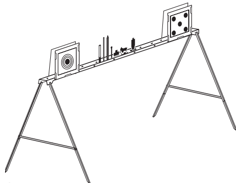
Стойка мишенная универсальная СМПУ-3
